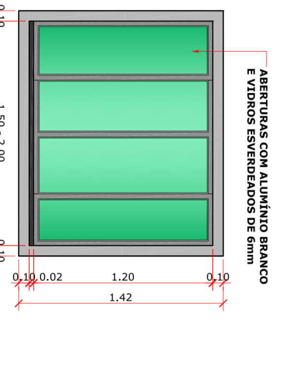
DETALHE 03 VERGA E CONTRA VERGA ESCALA RELATIVA
