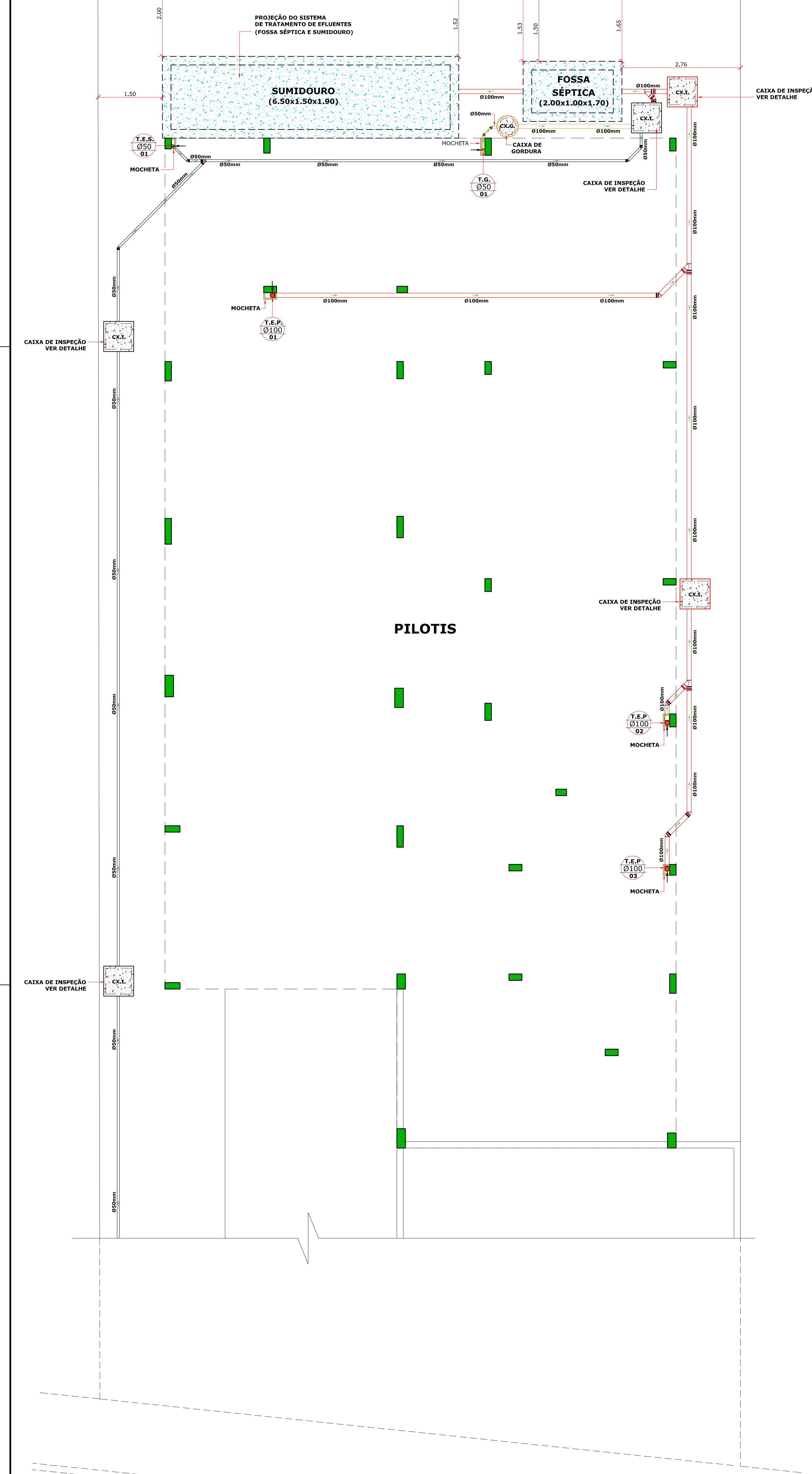
PLANTA BAIXA PAVIMENTO SUBSOLO (PILOTIS) ESCALA = 1 : 50
