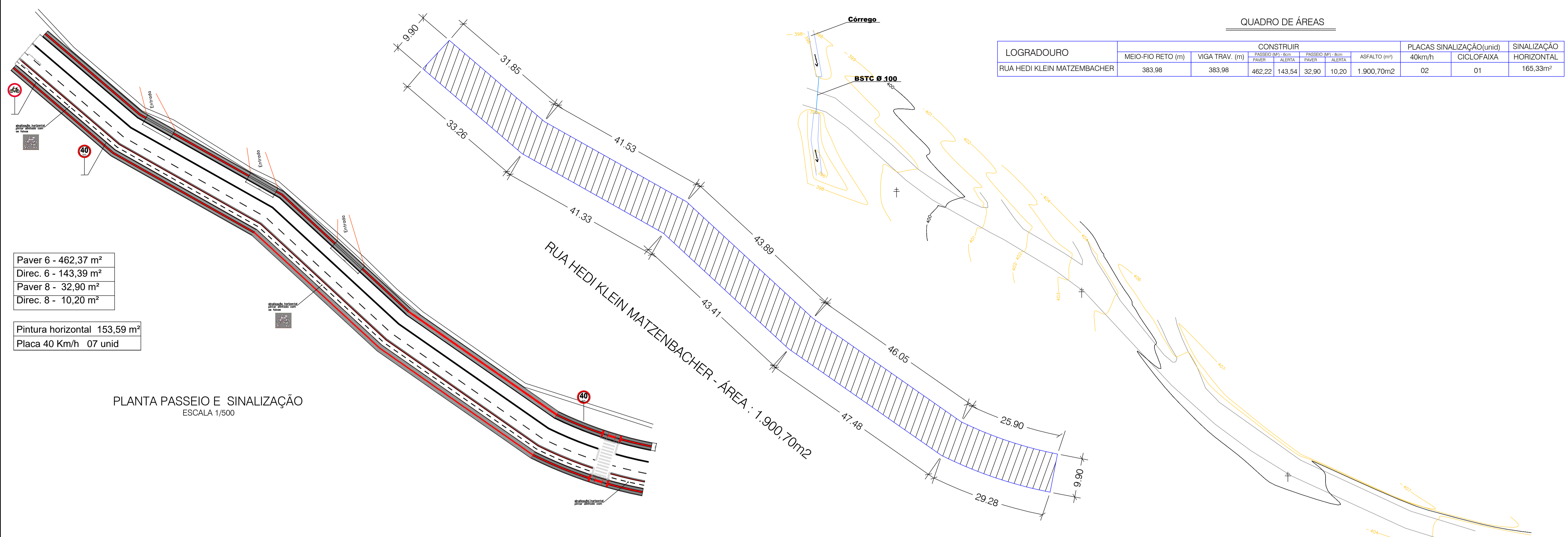
PLANTA CURVA DE NIVEIS ESCALA 1/500
