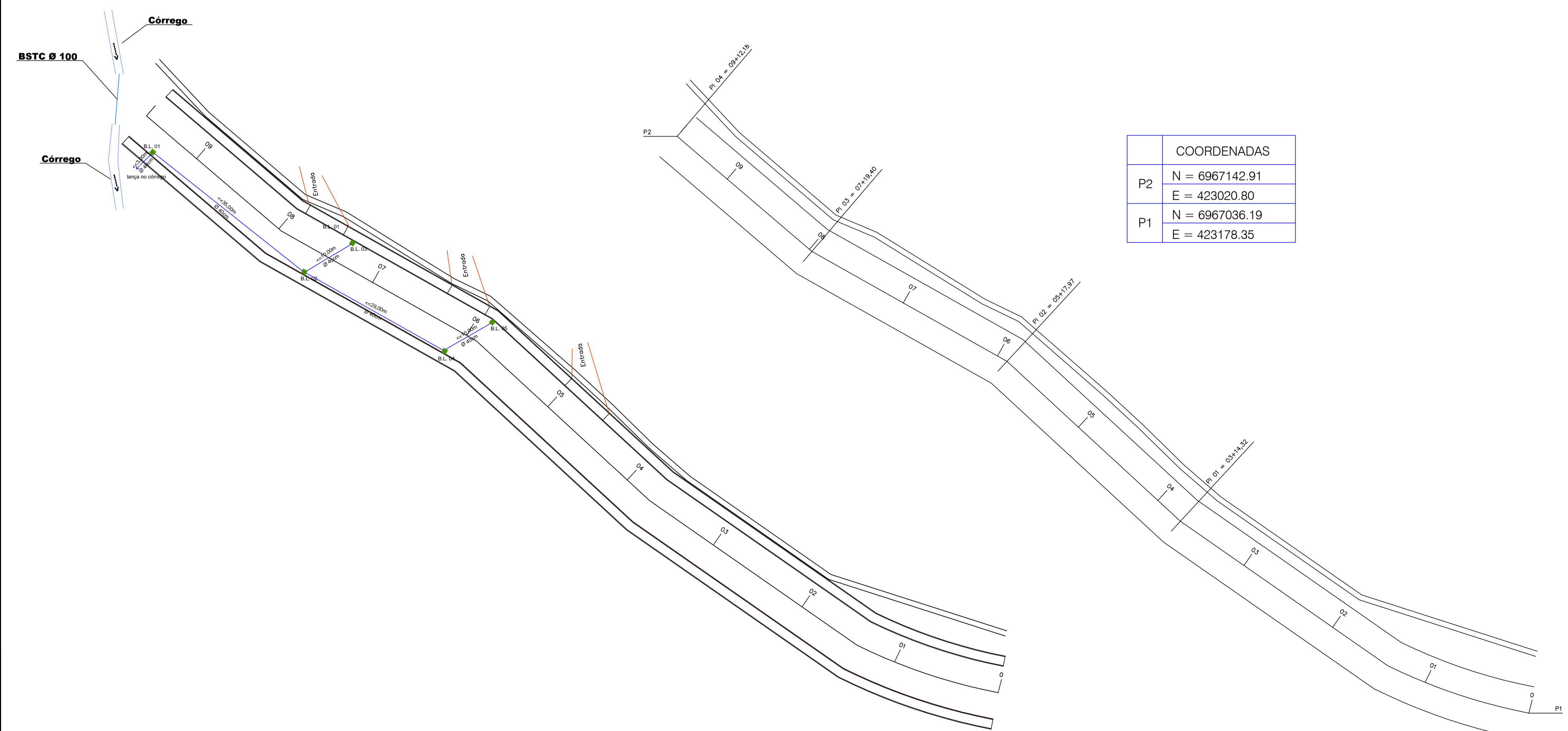
PLANTA DRENAGEM PLUVIAL ESCALA 1/500
