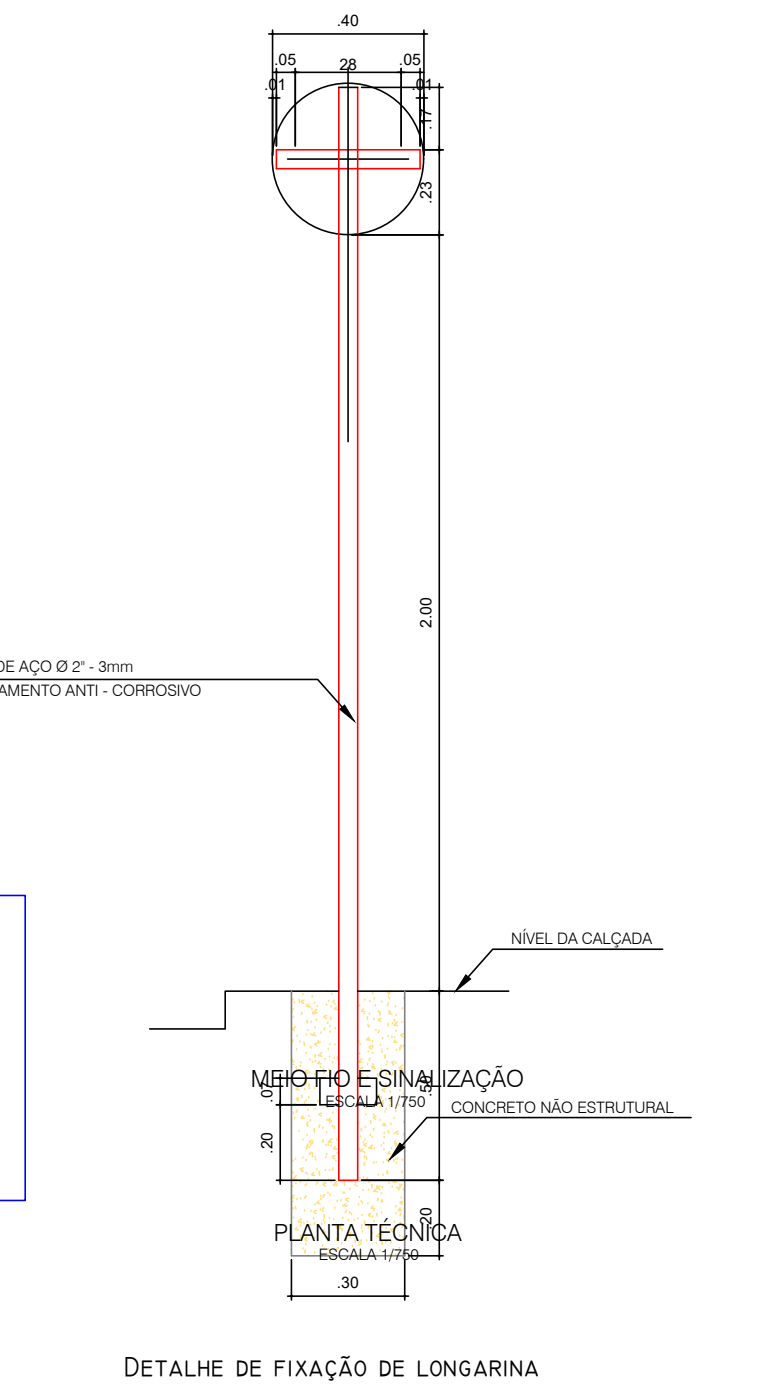
DETAILHE DE FIXAÇÃO DE LONGARINA
