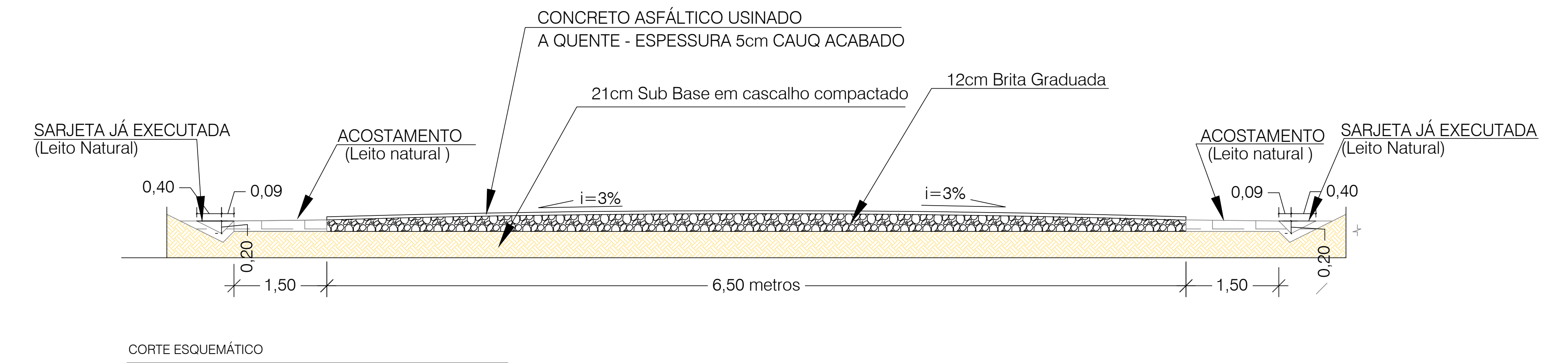
CORTE ESQUEMÁTICO
