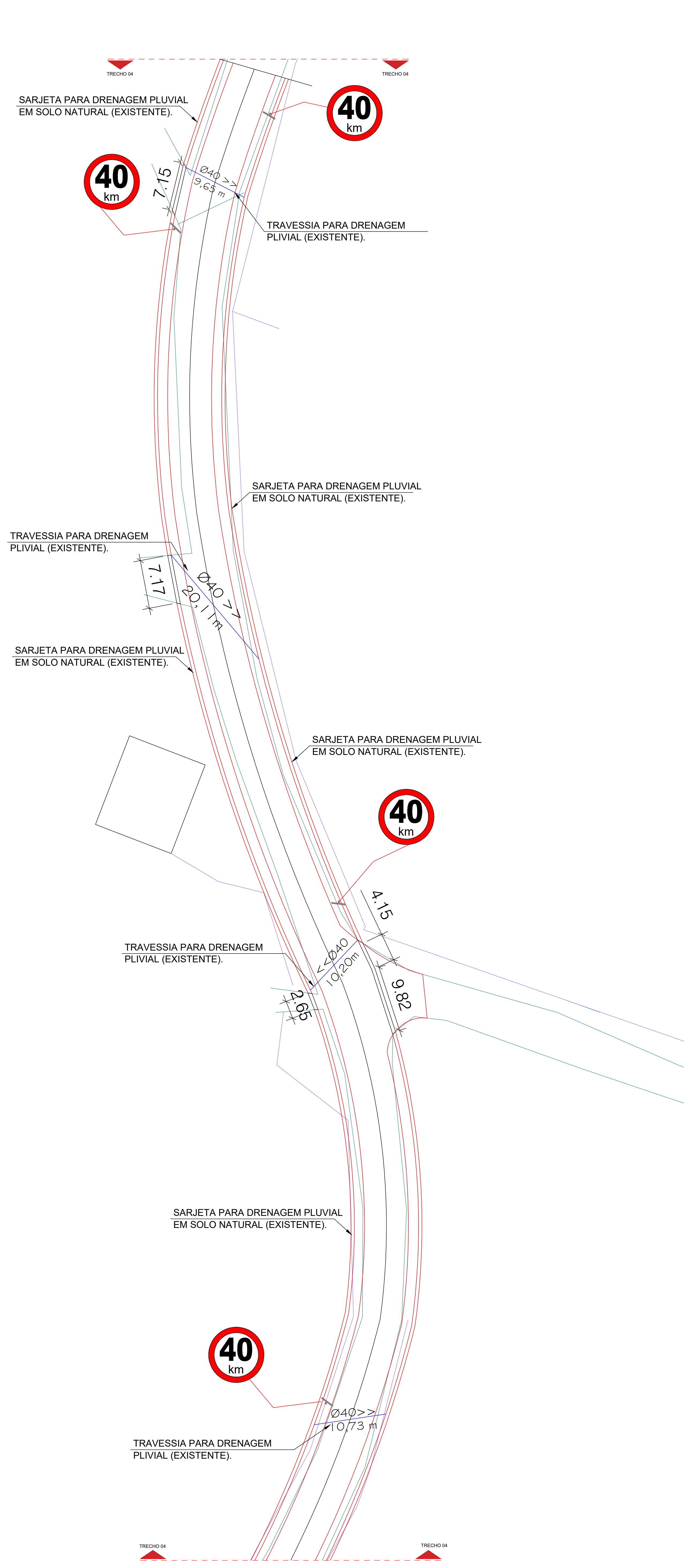
PROJETO PAVIMENTAÇÃO E SINALIZAÇÃO - TRECHO 04 ESCALA 1/300
