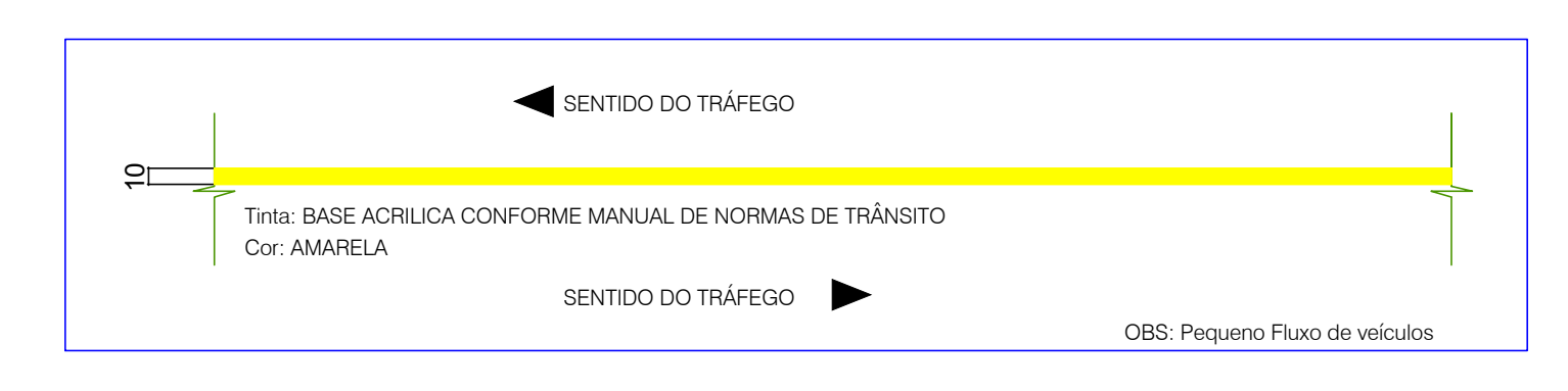
DETAILHE LINHA CONTÍNUA ESCALA: 1/100
