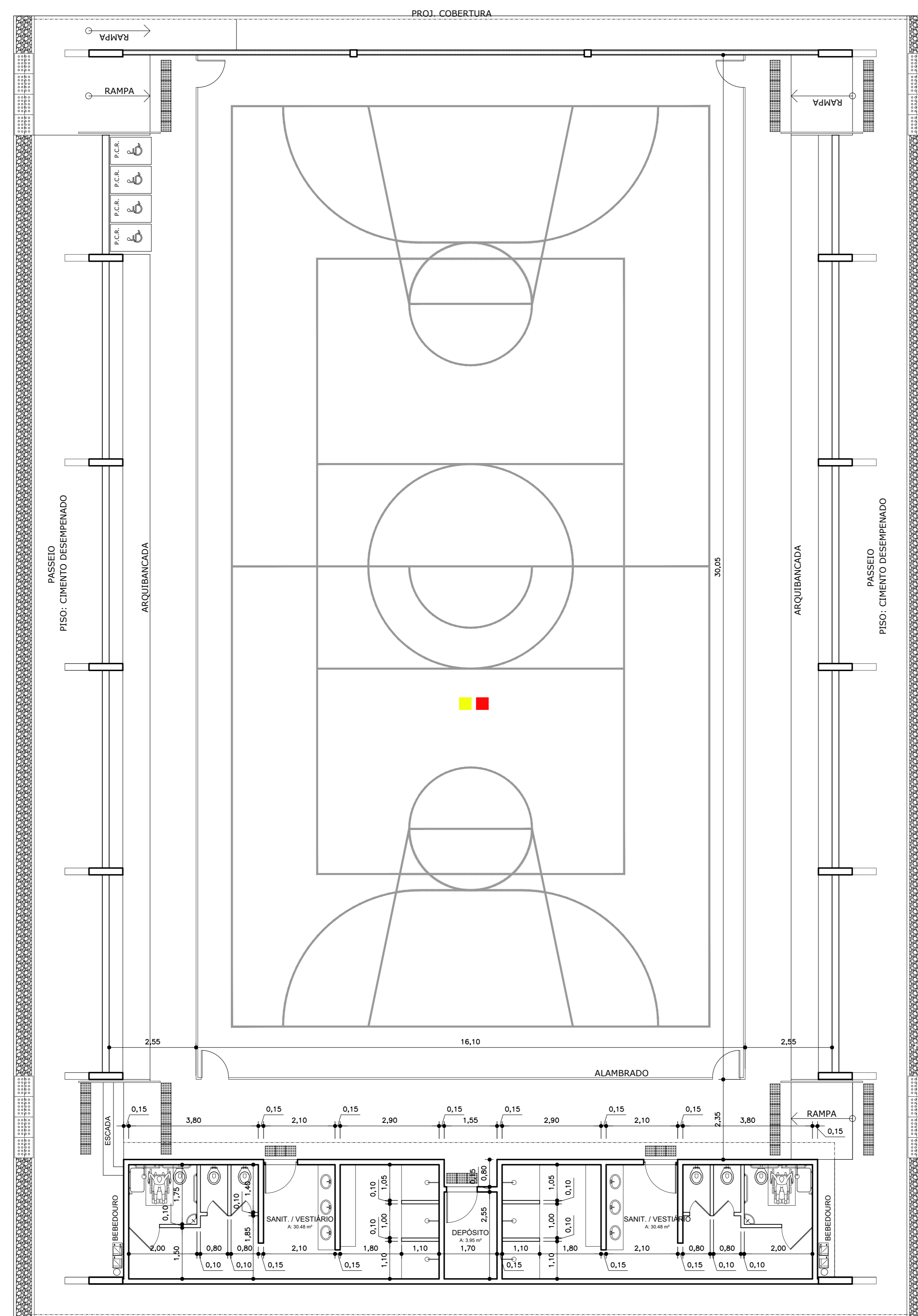
PLANTA BAIXA QUADRA POLIESPORTIVA Área: 778,74 m 2 Esc.: 1/75
