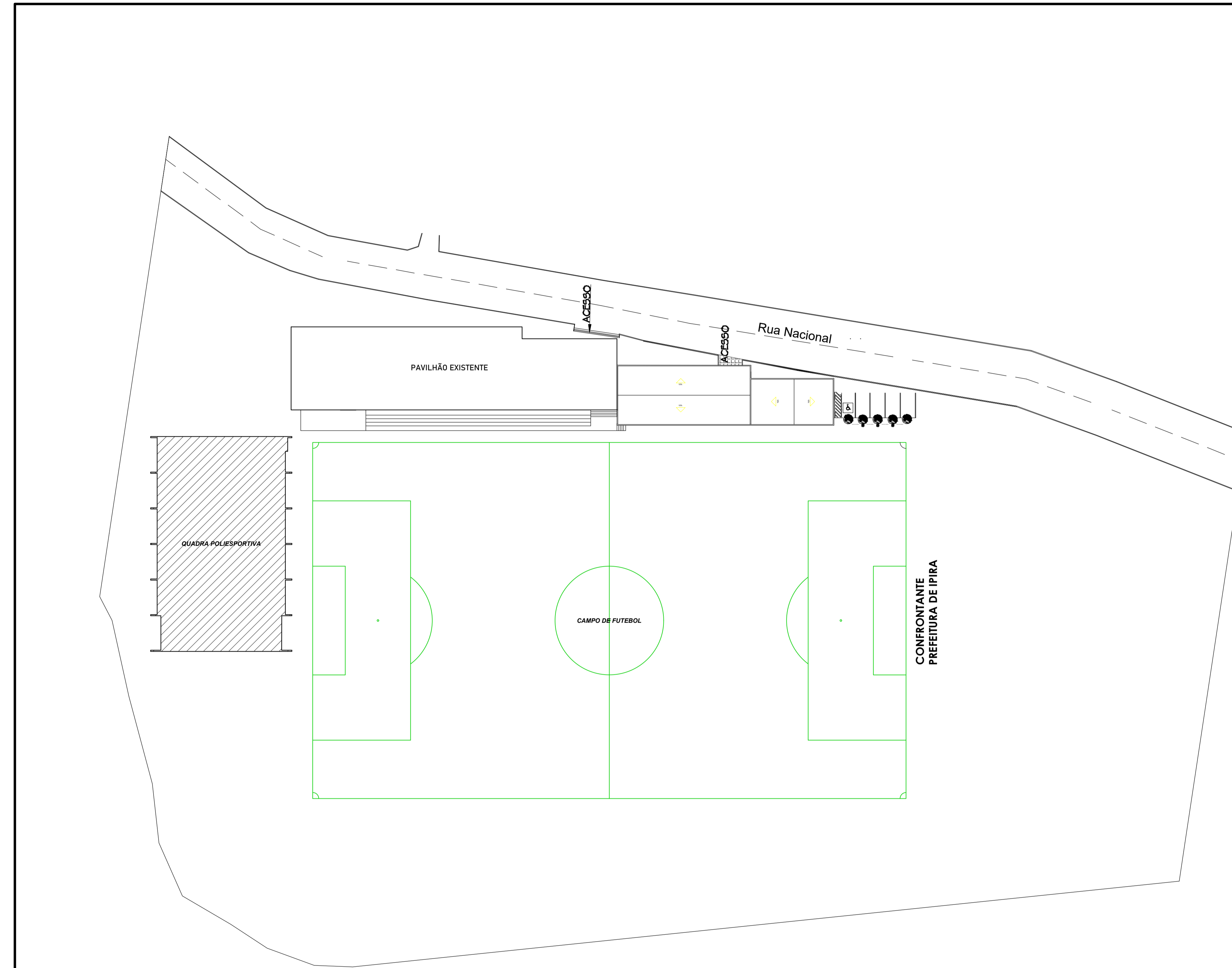
PLANTA DE LOCAÇÃO Esc.: ..... 1/400
