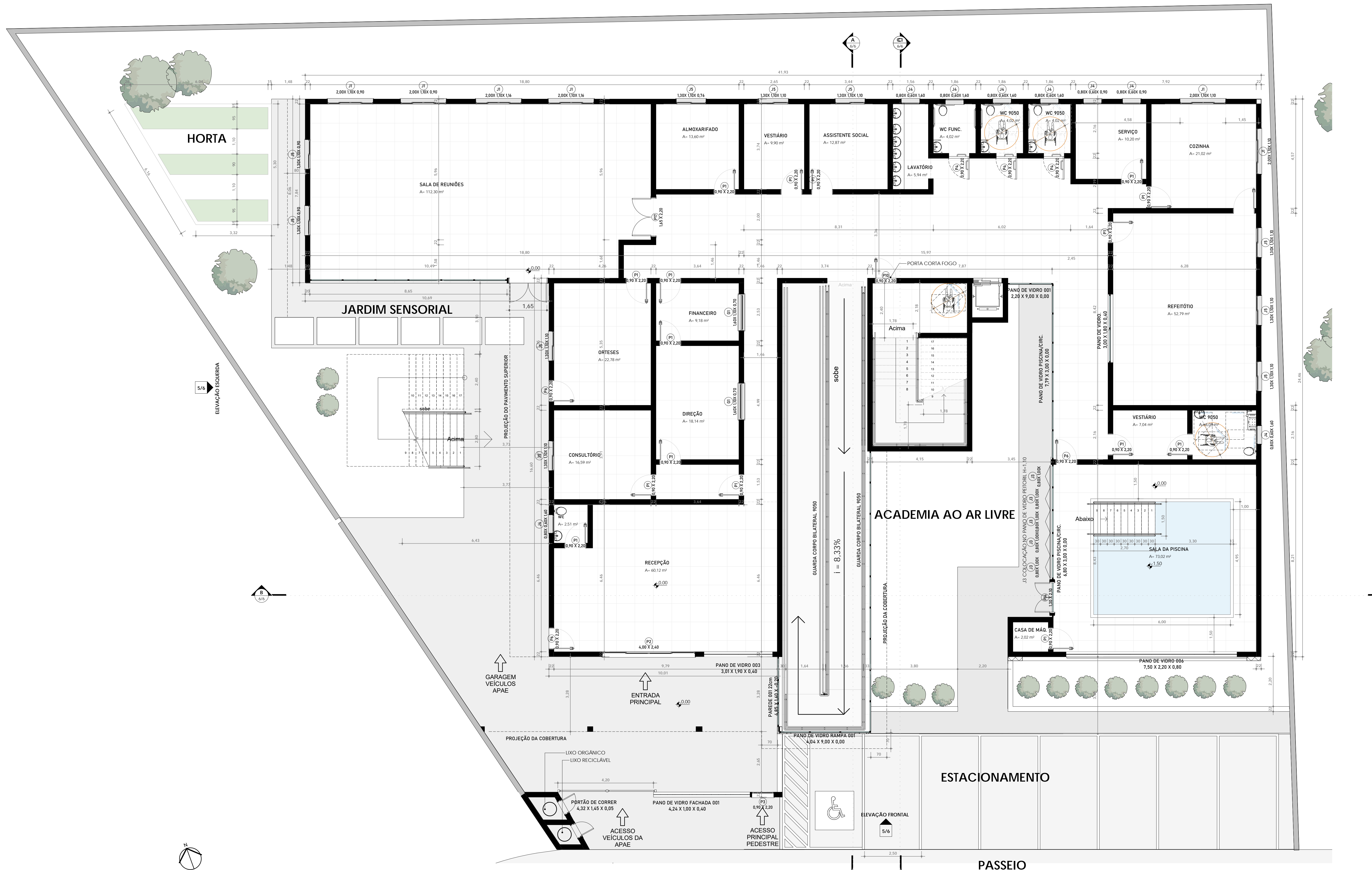
1 PLANTA BAIXA - PAVIMENTO TÉRREO ESC: 1 : 75
