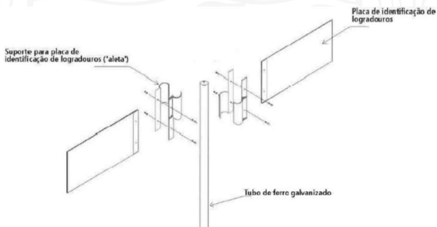
Figura 2 - Detalhe Fixação Placas de Identificação de Rua
