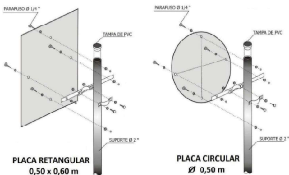
Figura 1 - Detalhe Fixação Placas
